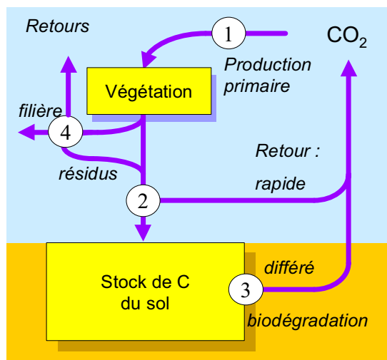
Figure 2-3. Problématique du stockage de carbone dans un agro- ou écosystème. Le stockage de \text{CO}_2 sous forme organique se pose en termes de flux \text{CO}_2 \rightarrow \text{C} organique et de durée de rétention sous forme organique. On distingue quatre postes affectant le stockage. (1) la production primaire : toutes choses étant égales par ailleurs, le stockage dans le sol sera d'autant plus élevé qu'elle est élevée. Son devenir se pose ensuite en termes de vitesses de retour à l'atmosphère. On distingue ici : (2) des alternatives au transfert au sol . C'est principalement la combustion, qui est un retour instantané. Concernant les déchets des filières de la production primaire, tels que lisiers et fumiers, composts, boues, on peut considérer en première approximation que leur devenir est le même que si les produits végétaux de départ étaient restés in situ. (3) les vitesse de biodégradation . Elles diffèrent le retour du carbone à l'atmosphère. Leur ralentissement provoque un stockage. (4) la gestion des filières et des durées de vie dans les filières ainsi que le retour différé et/ou le transfert des résidus de ces filières.
