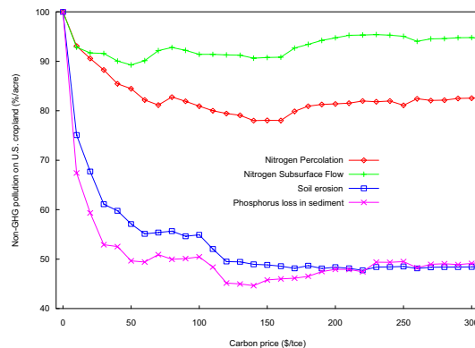
Figure 5-5. Impacts environnementaux des efforts de réduction du carbone émis par le secteur agricole des USA.
