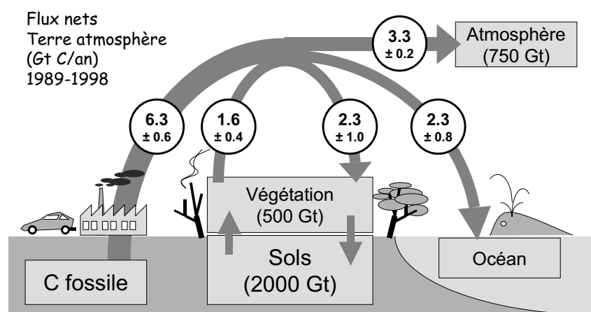
Figure 2-1. Cycle global du carbone : flux nets terre-atmosphère. La combustion de charbons et pétroles, avec la déforestation, injectent 7,9 \text{ GtC.an}^{-1} sous forme de CO 2 dans l'atmosphère. Or le réservoir atmosphérique augmente beaucoup moins. L'océan superficiel absorbe une partie de l'excédent. La végétation et les sols se comportent également comme un puits, situé essentiellement dans l'hémisphère nord. Ces flux nets sont petits par rapport aux échanges moyens annuels : environ 120 \text{ GtC.an}^{-1} entre biosphère continentale et atmosphère, environ 90 \text{ GtC.an}^{-1} entre océan et atmosphère. D'après GIEC 2001.
