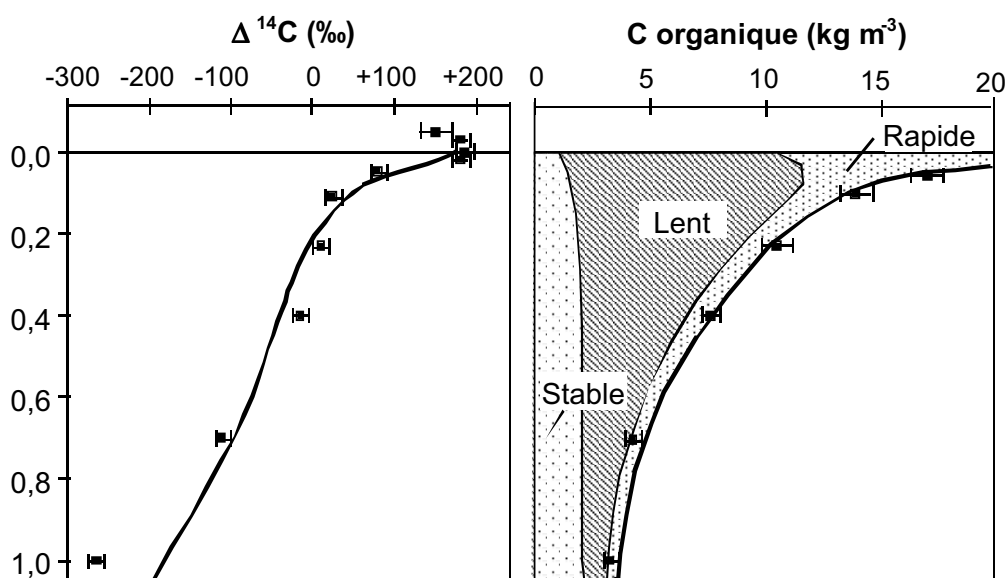
Figure 2-5. Répartition verticale des concentrations en carbone, de l'activité ^{14}\text{C} et des temps de résidence du carbone dans un sol forestier de l'Ile-de-France. La profondeur est exprimée en mètres.
