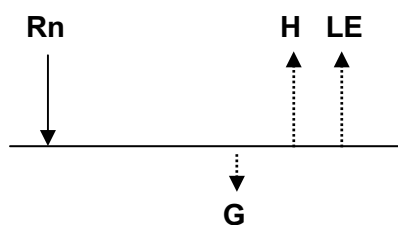
Figure A-4. Les composantes du bilan d'énergie (en journée).
