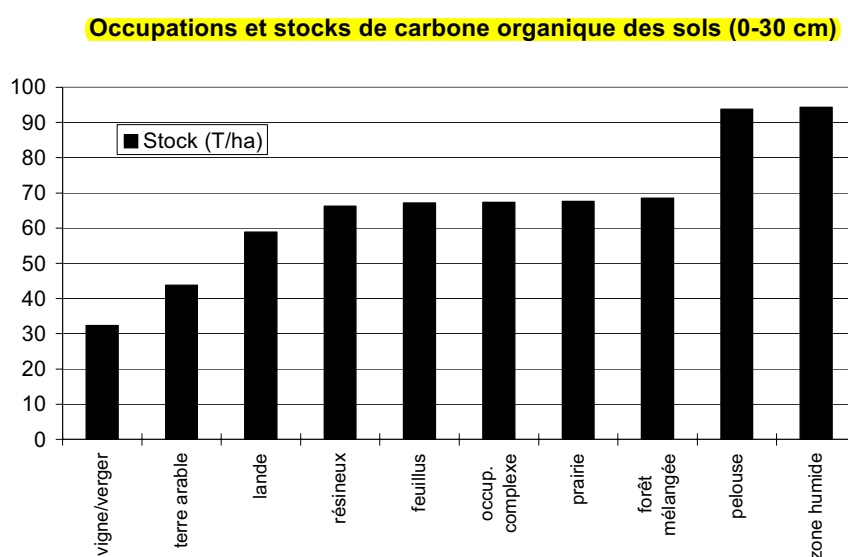
Figure 2-11. Stocks de carbone des sols et occupations du sol. Les stocks de carbone déterminés ne sont pas à l'équilibre avec l'occupation du sol, mais correspondent à des moyennes mesurées.
