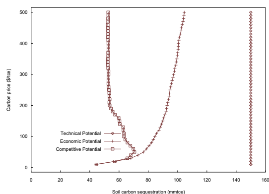
Figure 5-3. Courbe d'offre de stockage de carbone dans les sols agricoles aux Etats Unis. Sont incluses les variations de cultures traditionnelles et les prairies, ainsi que les variations de carbone dans les sols imputables à la transformation des cultures et prairies en forêt ou production de biocarburants.
